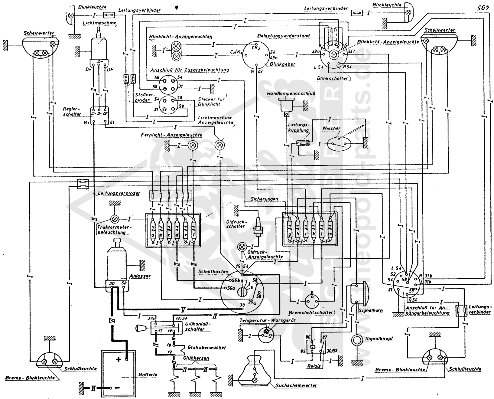
Schaltplan für Geräteträger F 230 GT
